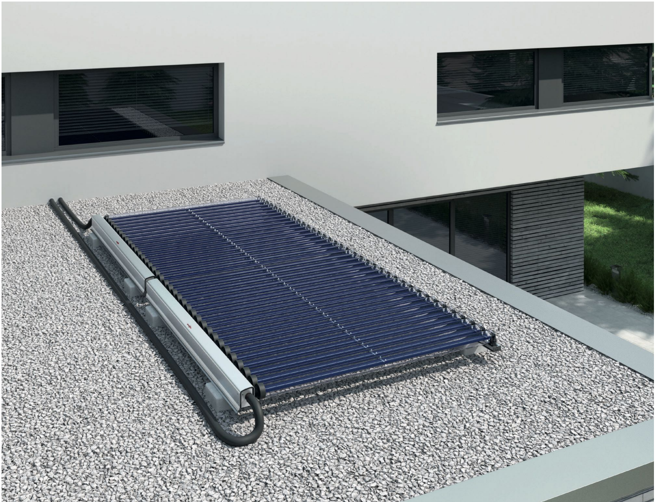
Beispiel für den Einsatz von Vitosol 200-TM Röhrenkollektoren mit Therm Protect
