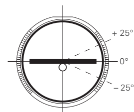
Einfache Installation und schnelle Absorberausrichtung durch Winkelanzeige an den Röhrenaufnahmen
